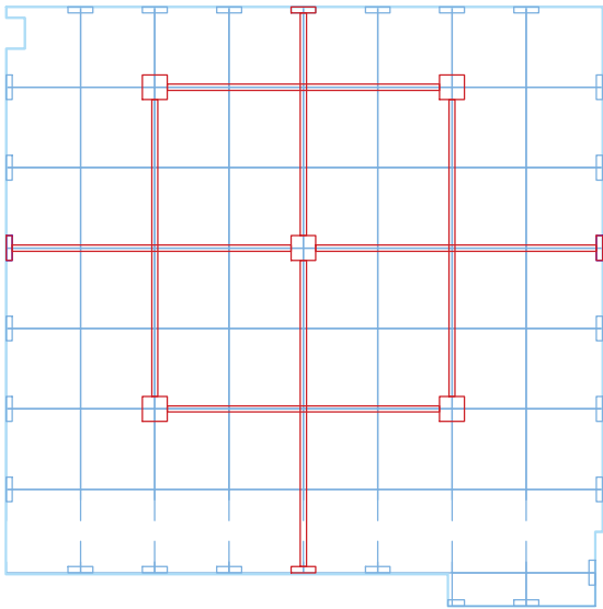
PLAN I PROFILEVE KOMPOZIMI 2
