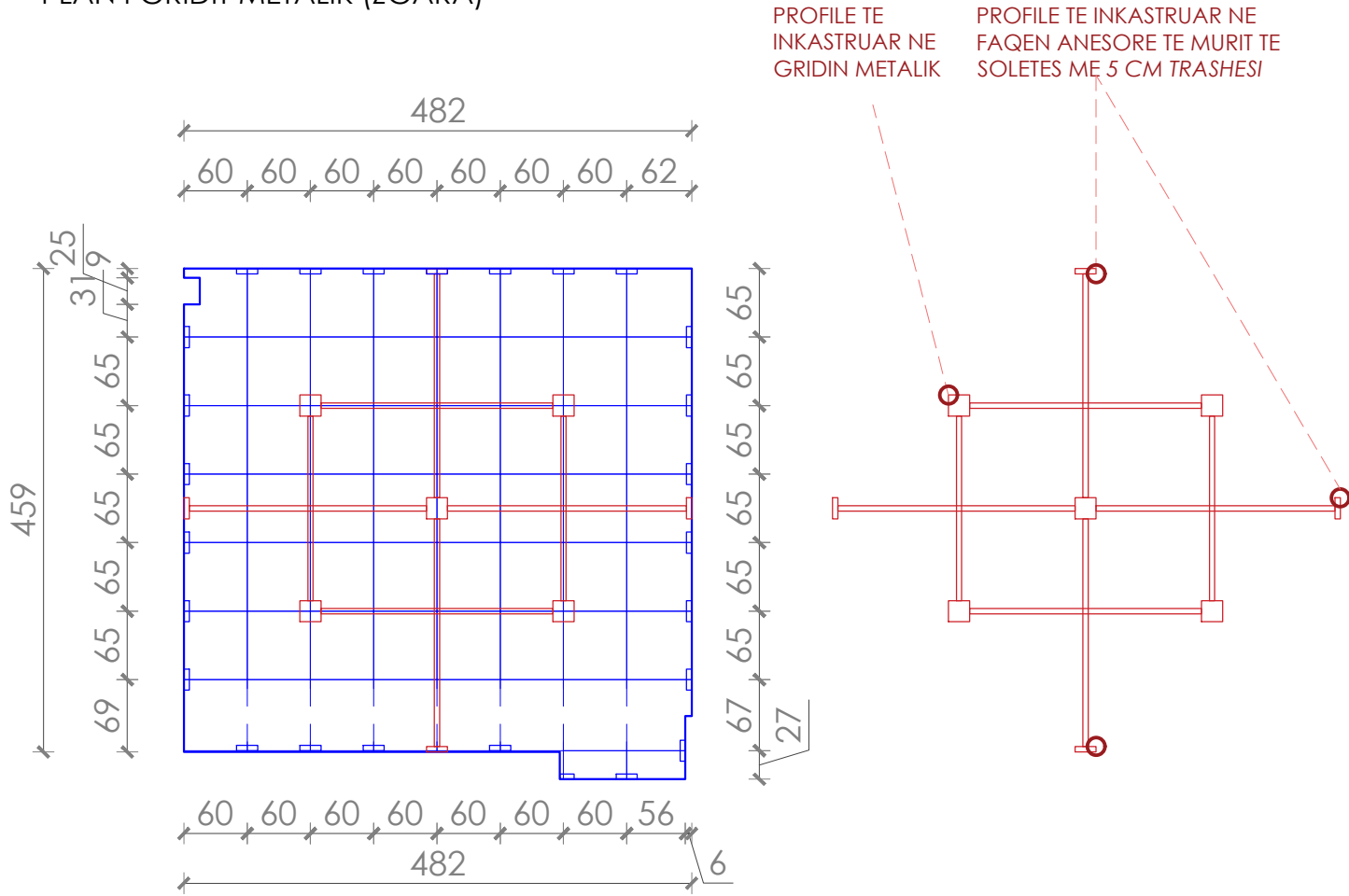
PLAN I GRIDIT METALIK (ZGARA)
