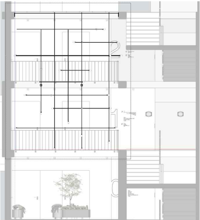
PAMJA A-A
